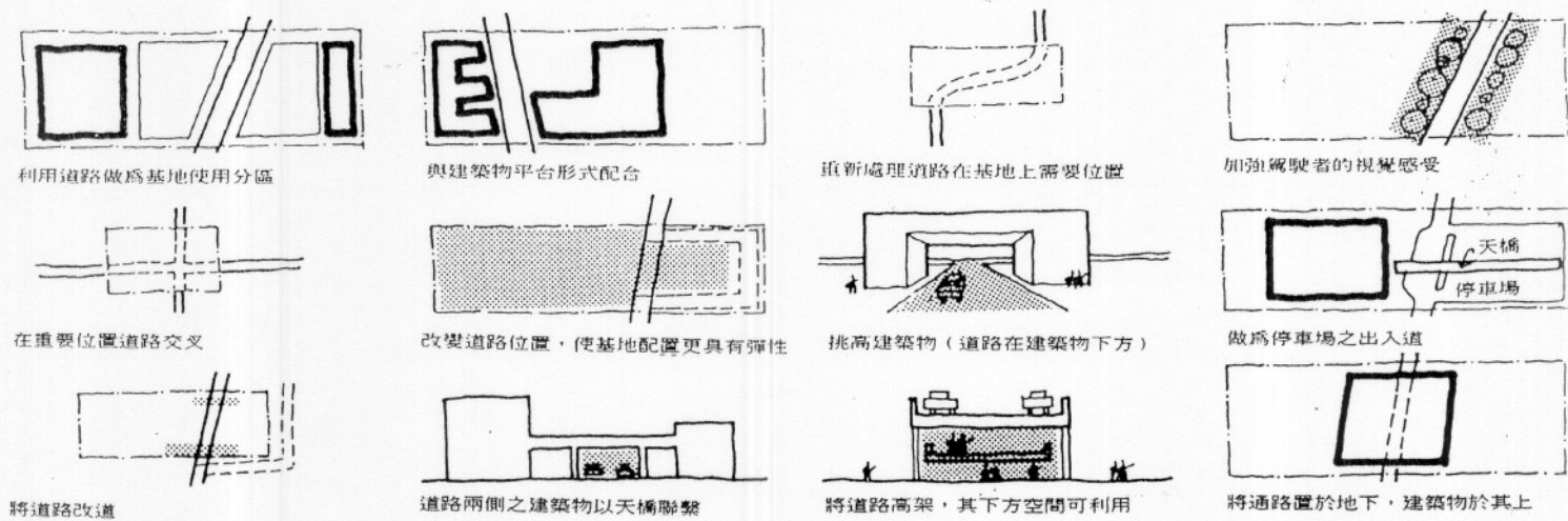
圖 1-2 基地內現有道路之處理
